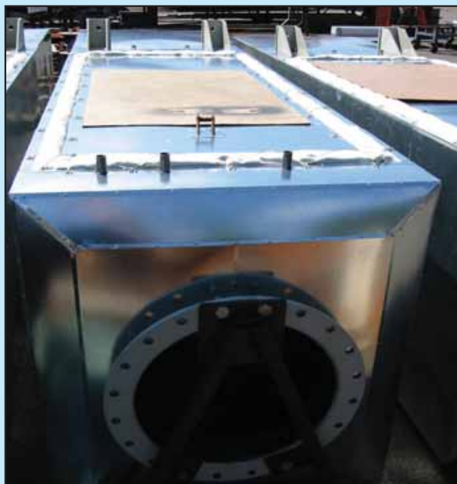
SCR-konverteren produseres i stål. Etterpå blir den isolert. I konverteren plasseres keramiske elementer som renser ved hjelp av urea.
